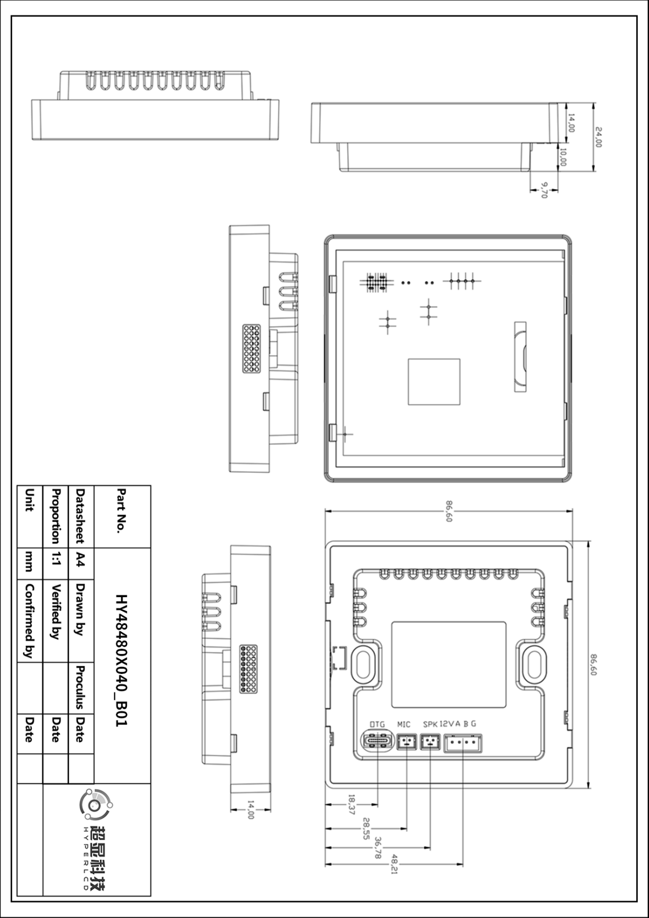
产品尺寸图（产品包含外壳）
